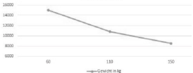
Lastendiagramm
